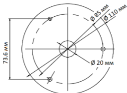
Рисунок 2-5 Шаблон крепления
