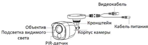
Рисунок 1-1 Камера I типа
